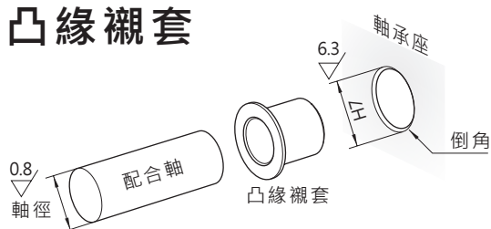
a b 外徑倒角
